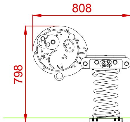
ALZADO
