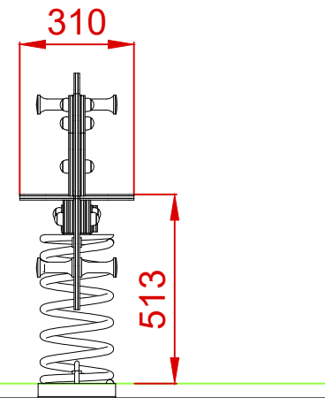
PERFIL
