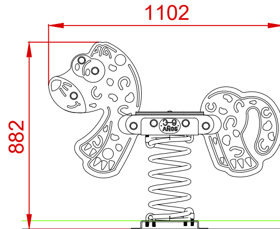
ALZADO
