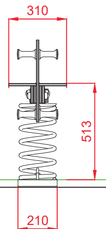
PERFIL
