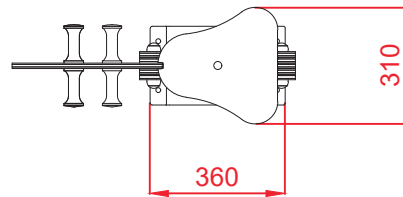
PLANTA
