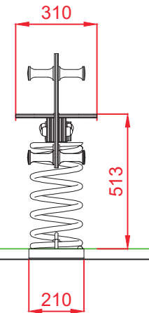
PERFIL
