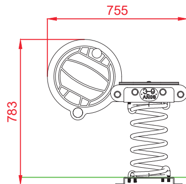
ALZADO
