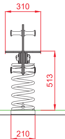
PERFIL
