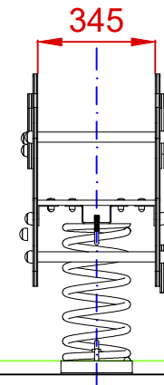
PERFIL
