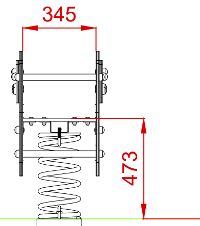
PERFIL
