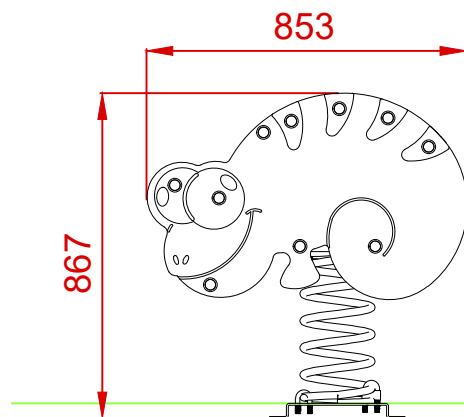
ALZADO
