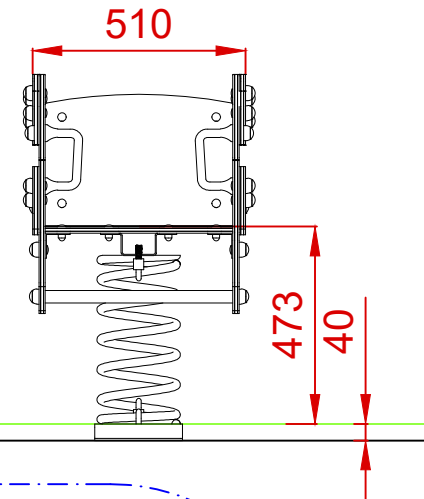
PERFIL
