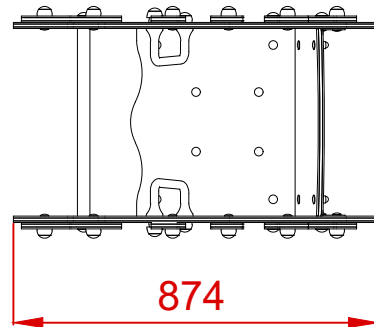
PLANTA
