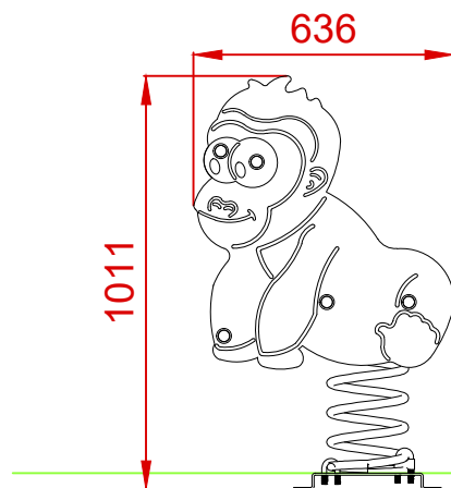
ALZADO
