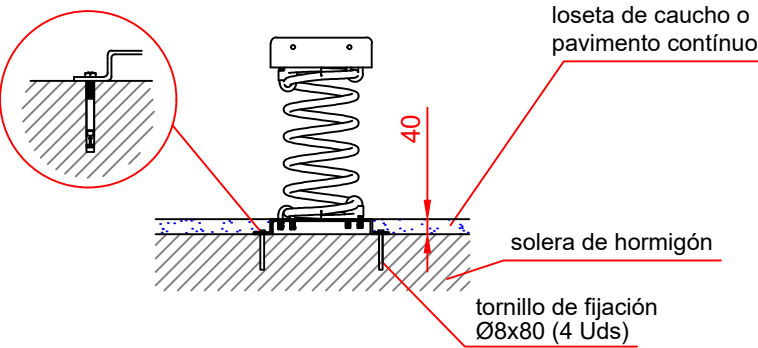
Detalle se sujeción de espirro metálico
