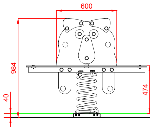
ALZADO
