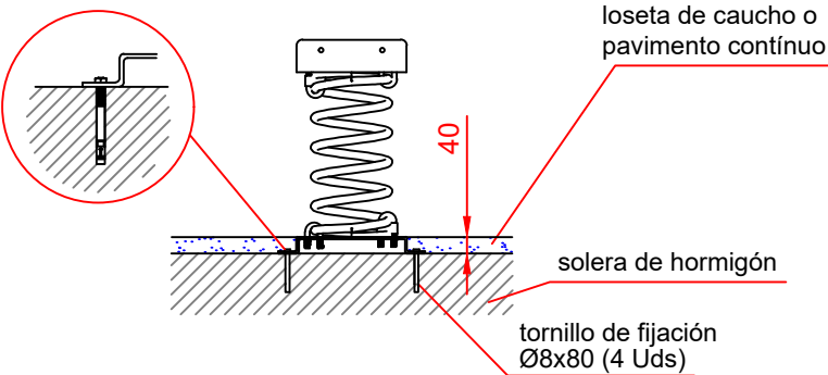
Detalle se sujeción de espirro metálico
