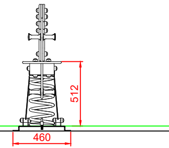
PERFIL
