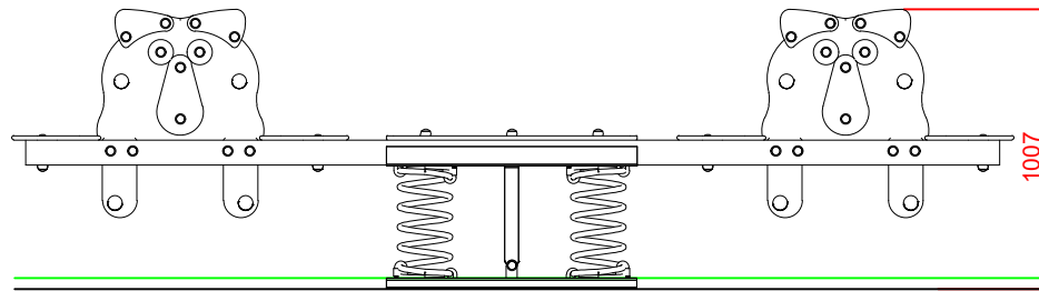
ALZADO
