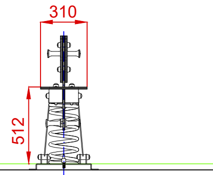
PERFIL
