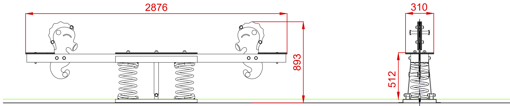
ALZADO
