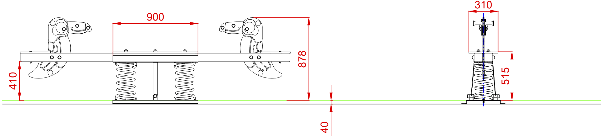
ALZADO
