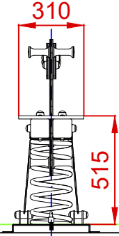
PERFIL
