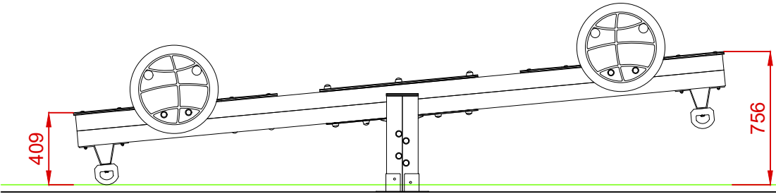
ALZADO POSICION DE APOYO
