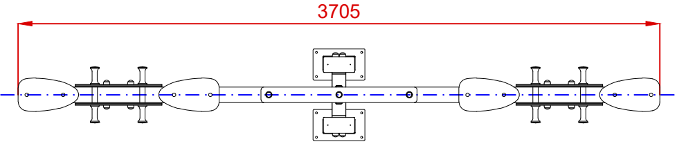
PLANTA
