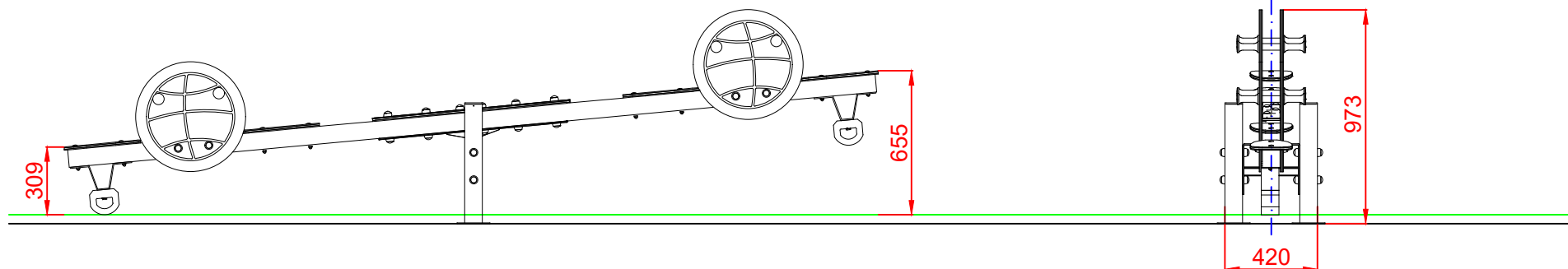
ALZADO
