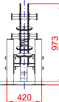
PERFIL
