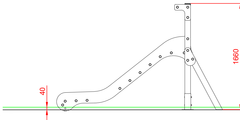
ALZADO
