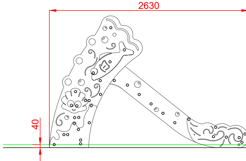
ALZADO
