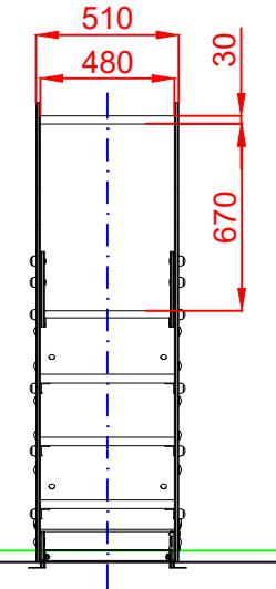
PERFIL
