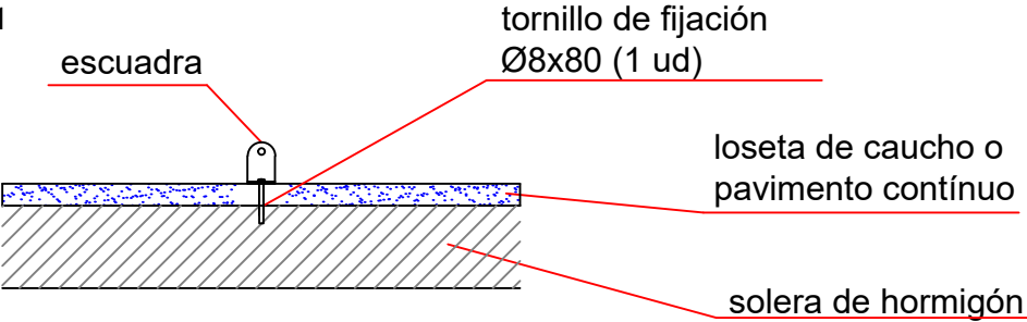
ESQUEMA DE CIMENTACIÓN EN HORMIGÓN E: 2/1
