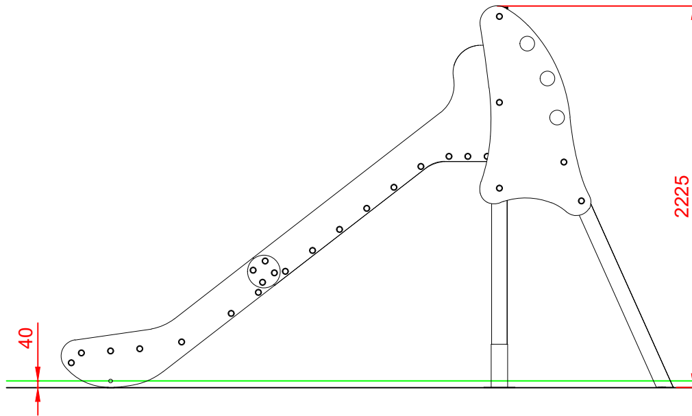
ALZADO
