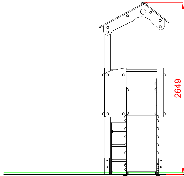
PERFIL DERECHO
