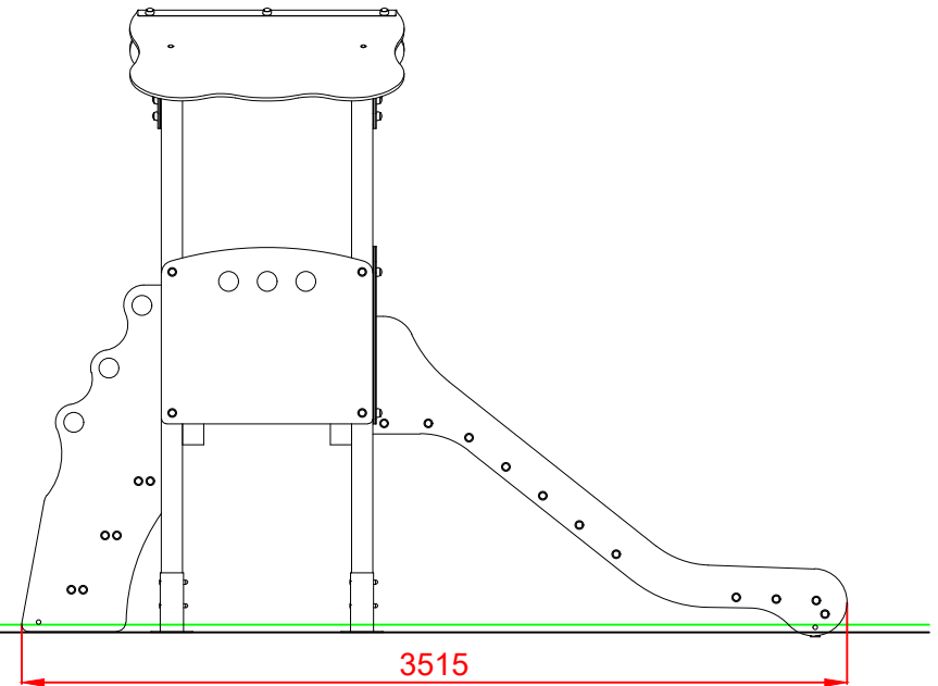
ALZADO
