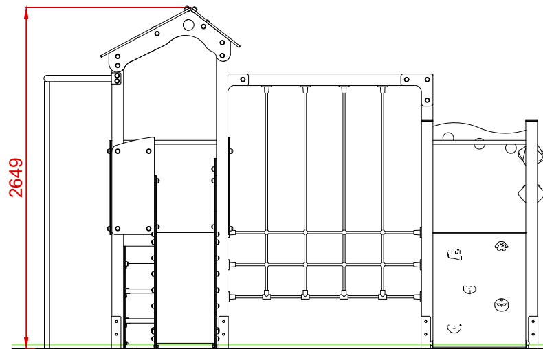
ALZADO
