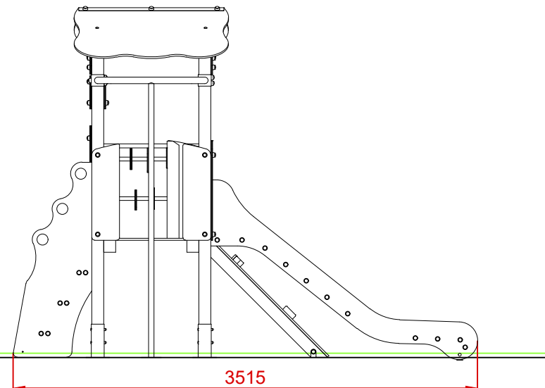
PERFIL IZQUIERDO
