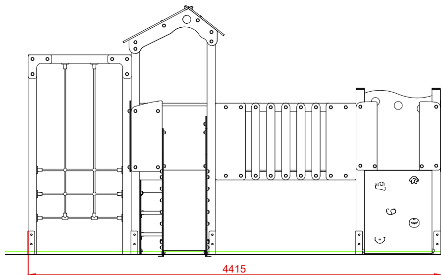
ALZADO
