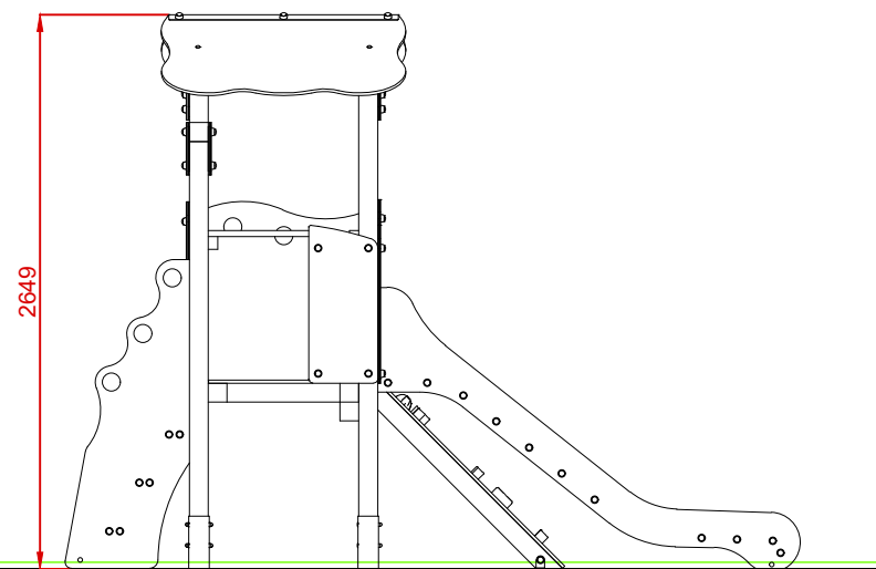
PERFIL IZQUIERDO
