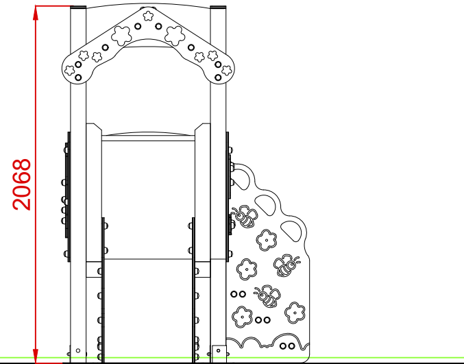
PERFIL IZQUIERDO
