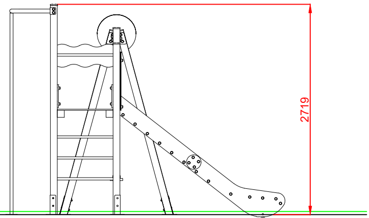
PERFIL IZQUIERDO
