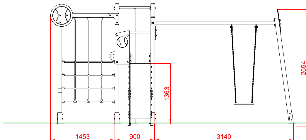
ALZADO
