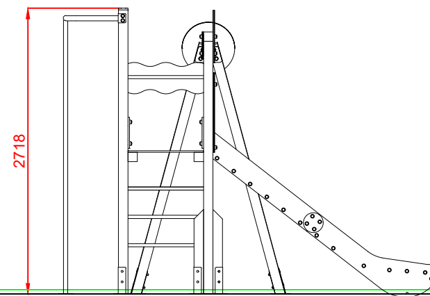
PERFIL IZQUIERDO
