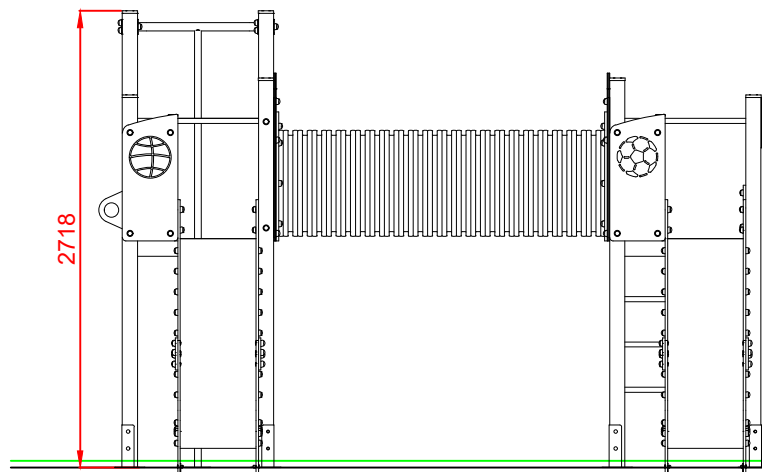
ALZADO
