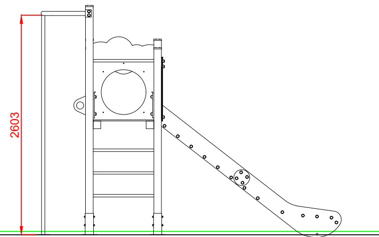
PERFIL IZQUIERDO
