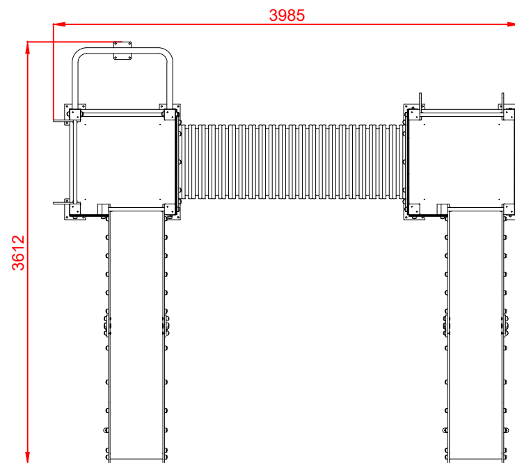
PLANTA
