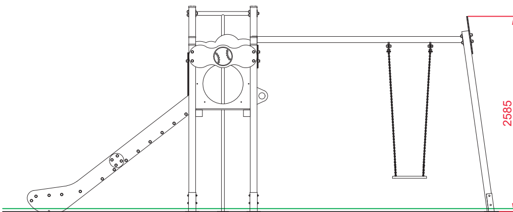
ALZADO
