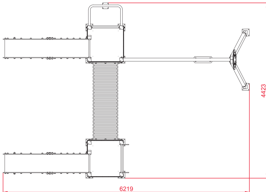
PLANTA
