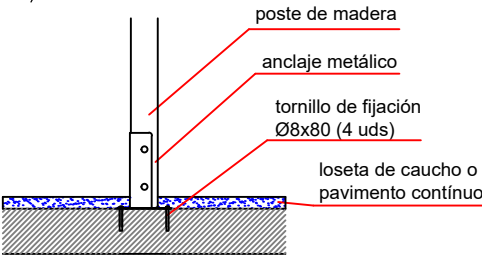
ESQUEMA DE CIMENTACIÓN EN HORMIGÓN E: 2/1
