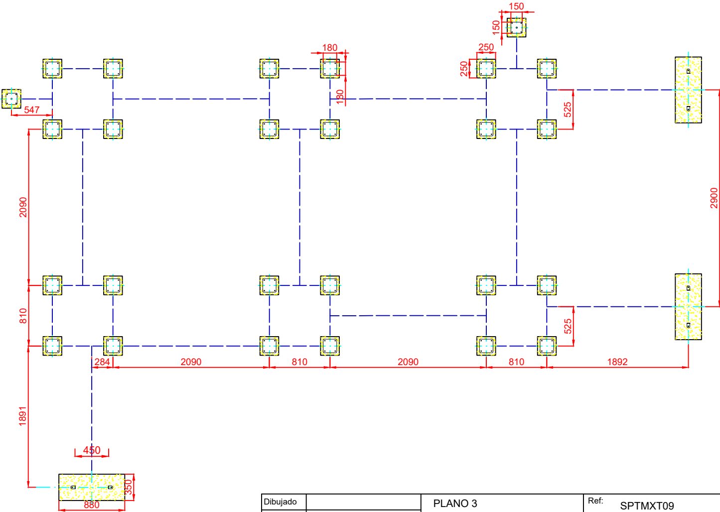
PLANTA CIMENTACIÓN
