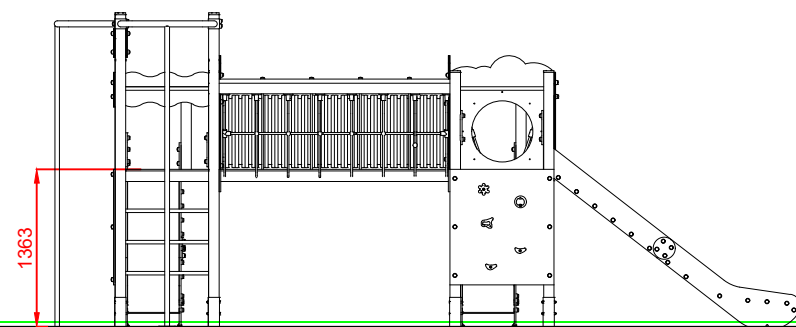
PERFIL IZQUIERDO
