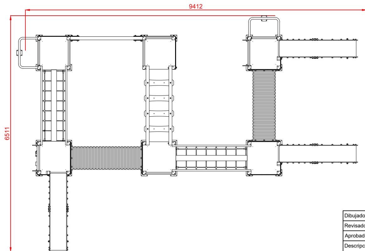
PLANTA
