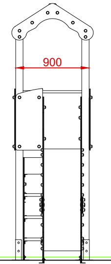
PERFIL
