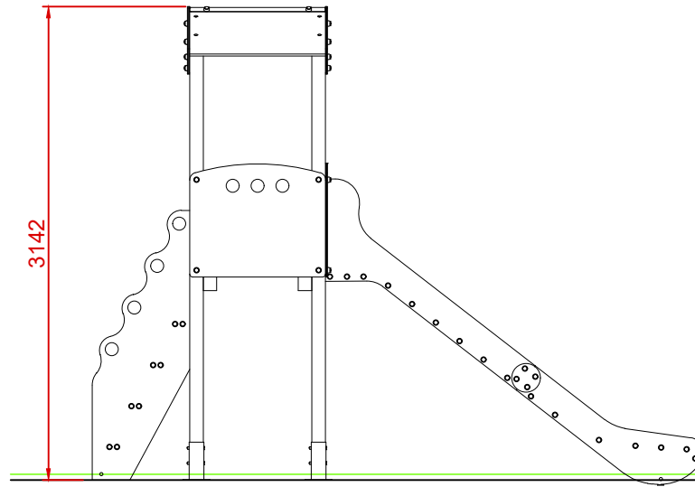
ALZADO
