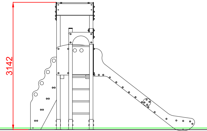
PERFIL
