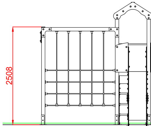
ALZADO
