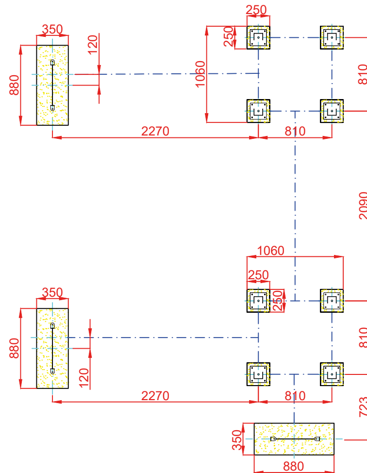
PLANTA DE CIMENTACIÓN
