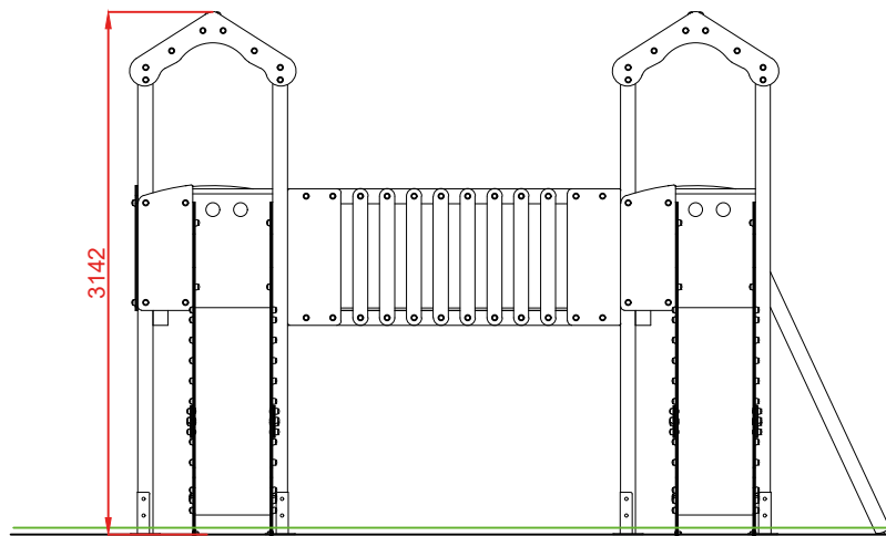
ALZADO
