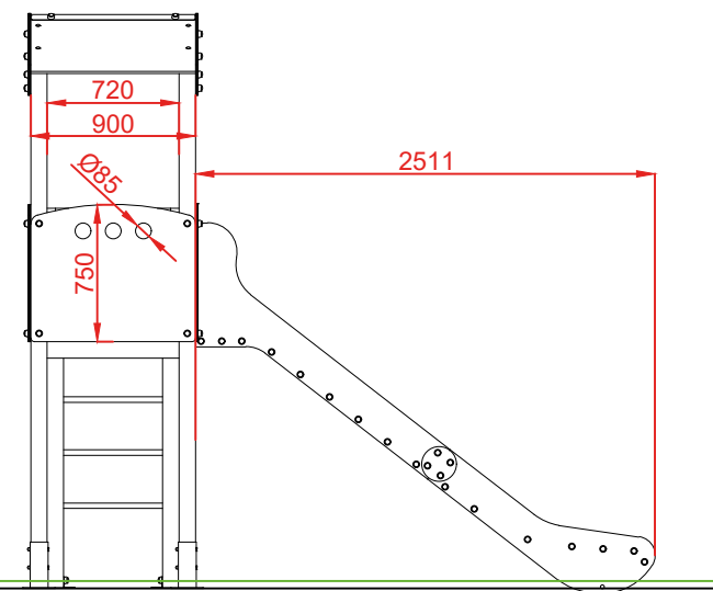
PERFIL IZQUIERDO
