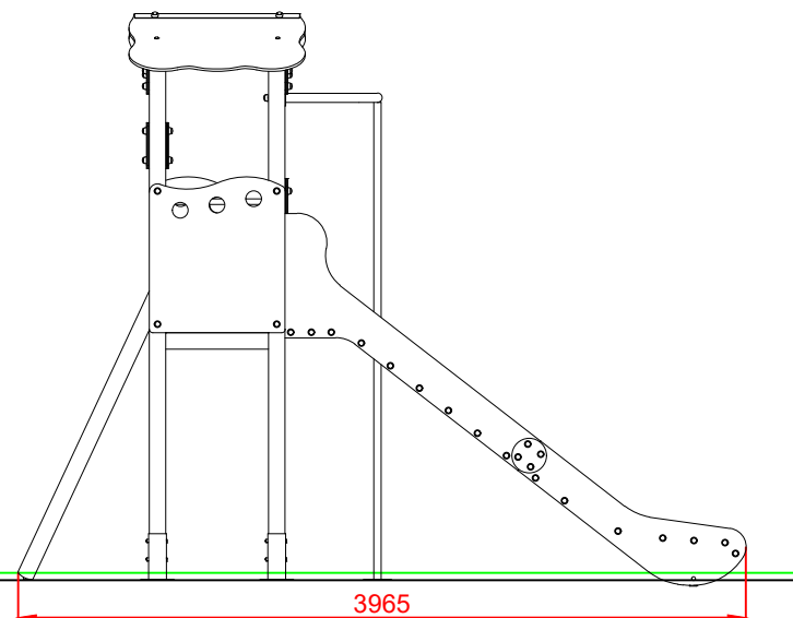
PERFIL IZQUIERDO
