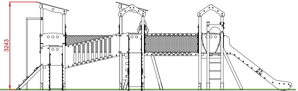
PERFIL IZQUIERDO
