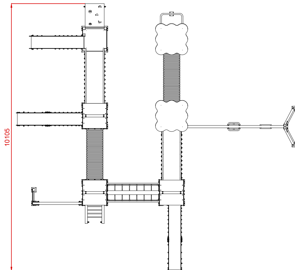
PLANTA
