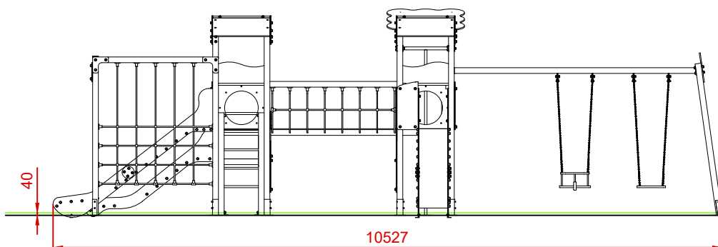
ALZADO
