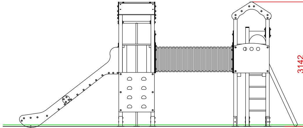
ALZADO
