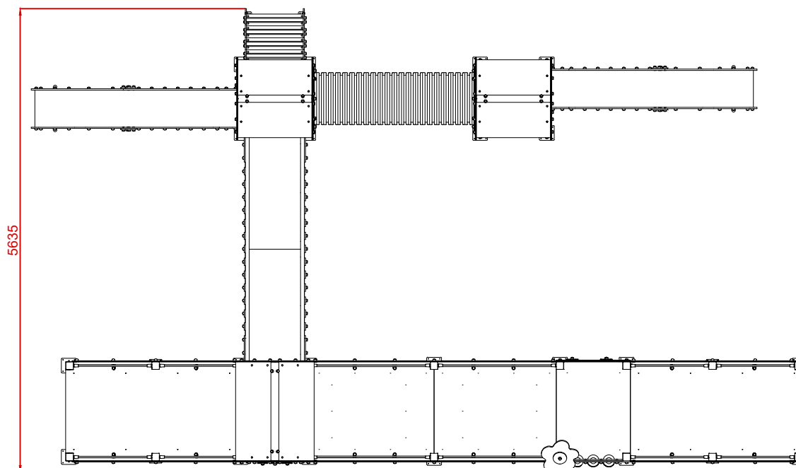
PLANTA
