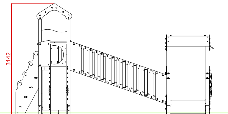
PERFIL IZQUIERDO
