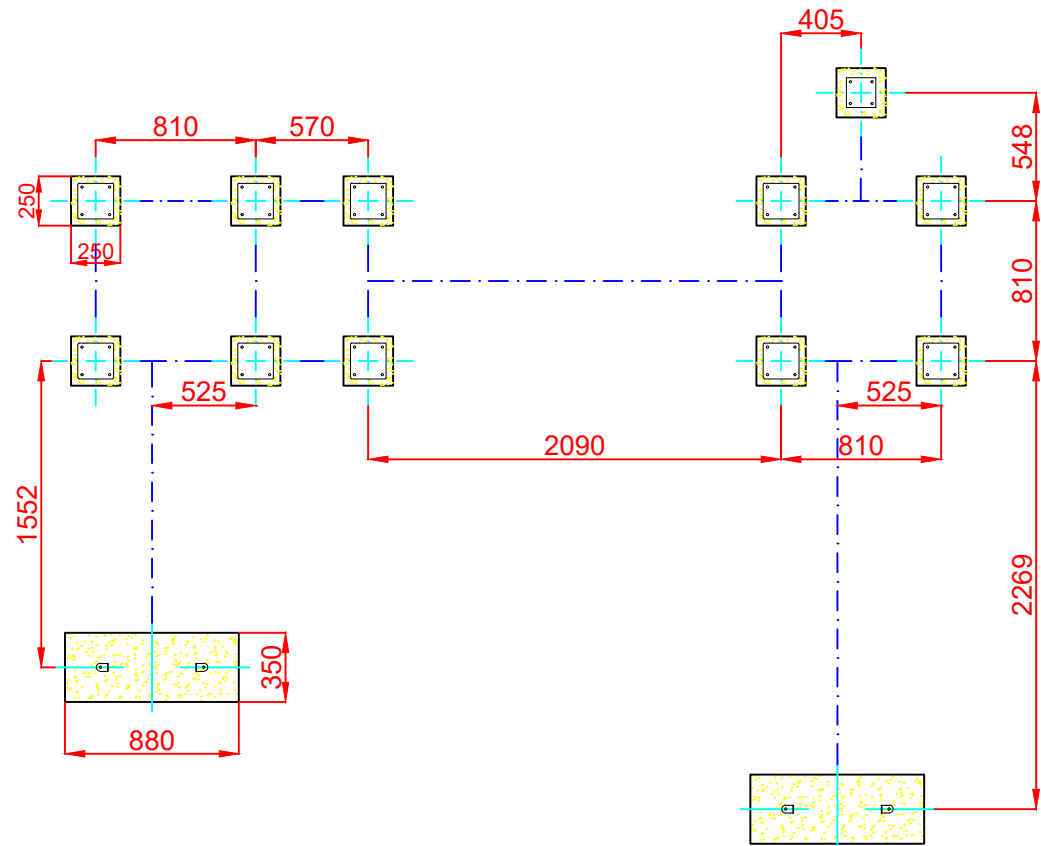
PLANTA CIMENTACIÓN
