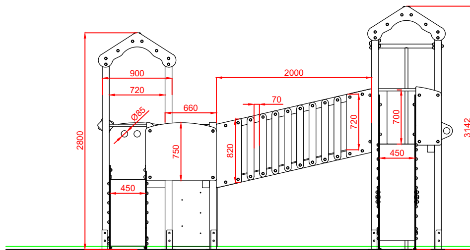
ALZADO
