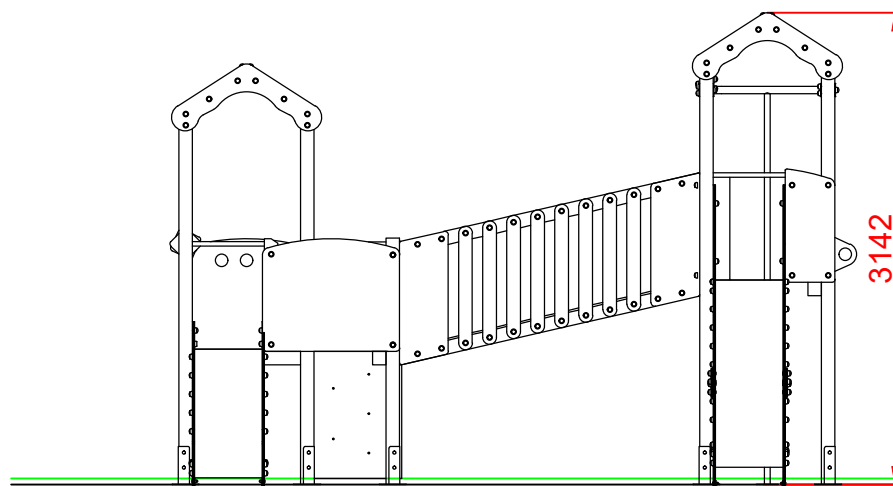
ALZADO
