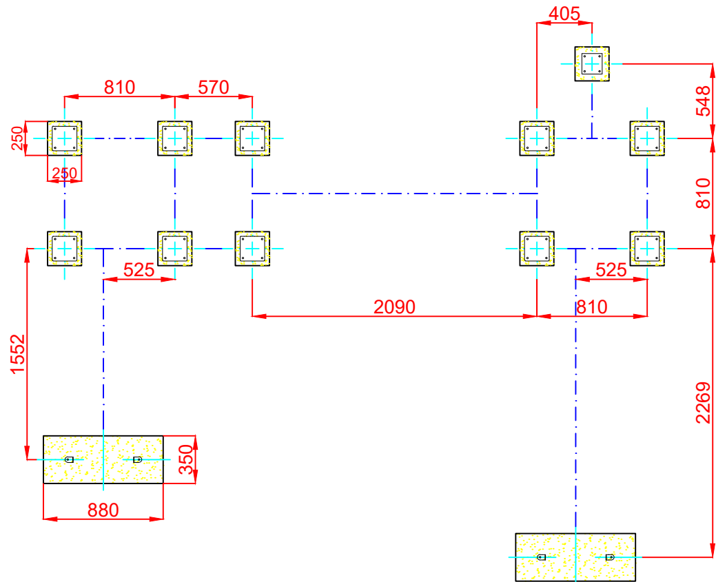
PLANTA CIMENTACIÓN
