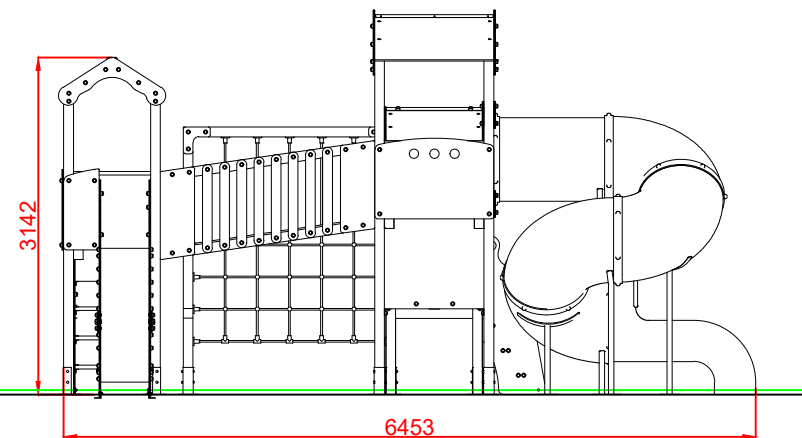
PERFIL DERECHO
