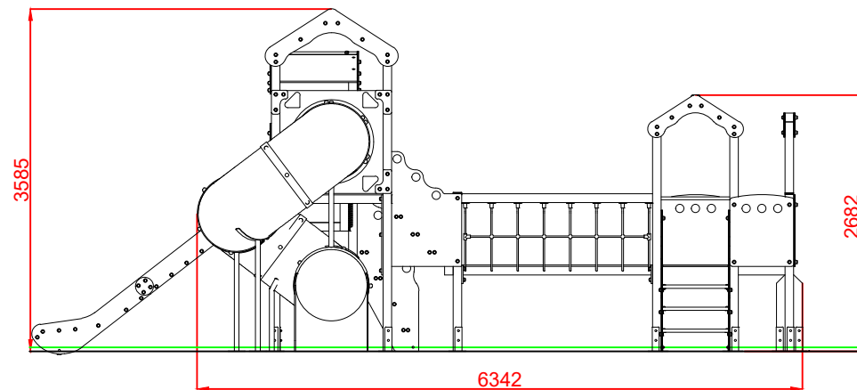
ALZADO
