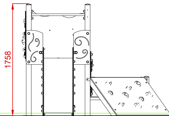
PERFIL IZQUIERDO
