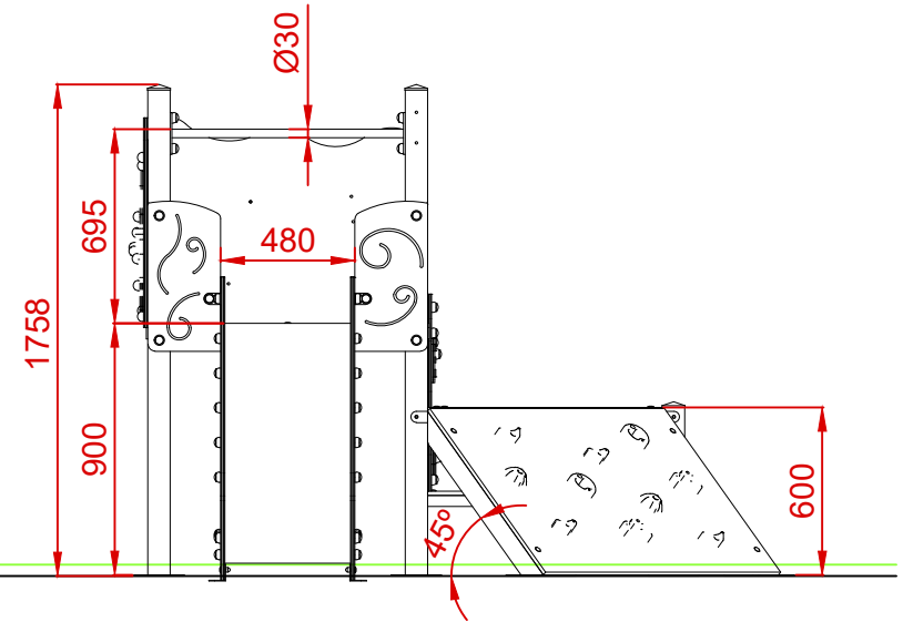
PERFIL IZQUIERDO
