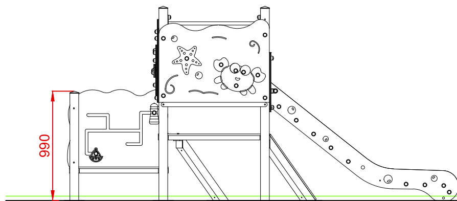
ALZADO
