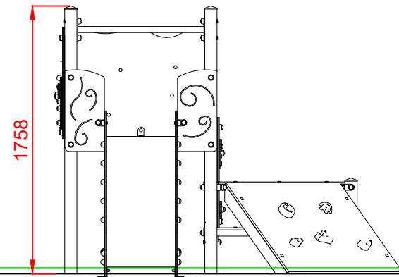
PERFIL IZQUIERDO
