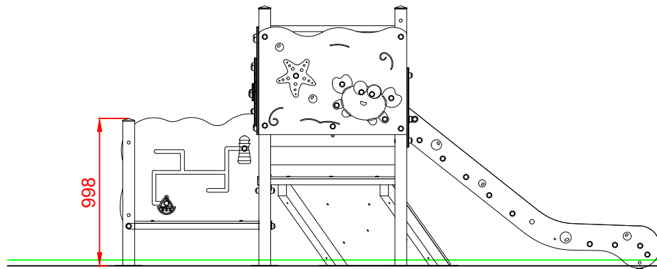
ALZADO
