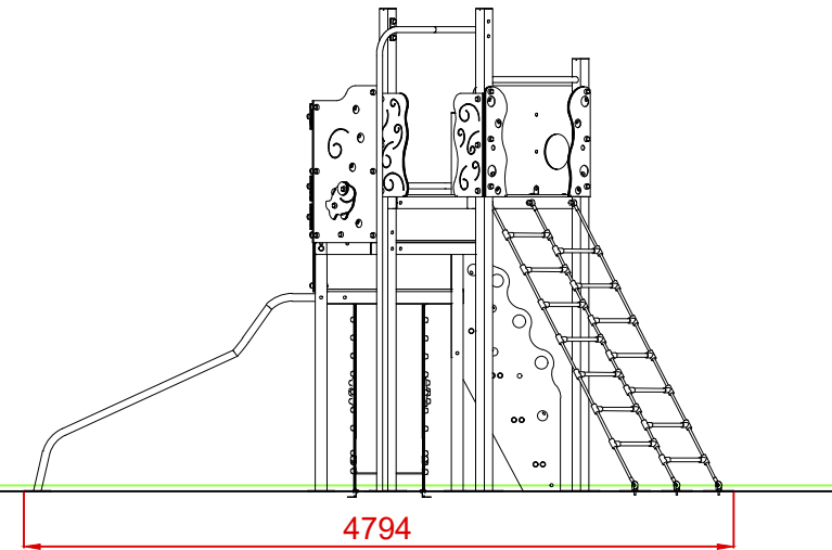
PERFIL IZQUIERDO
