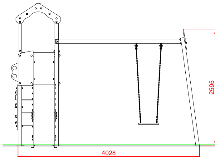
ALZADO
