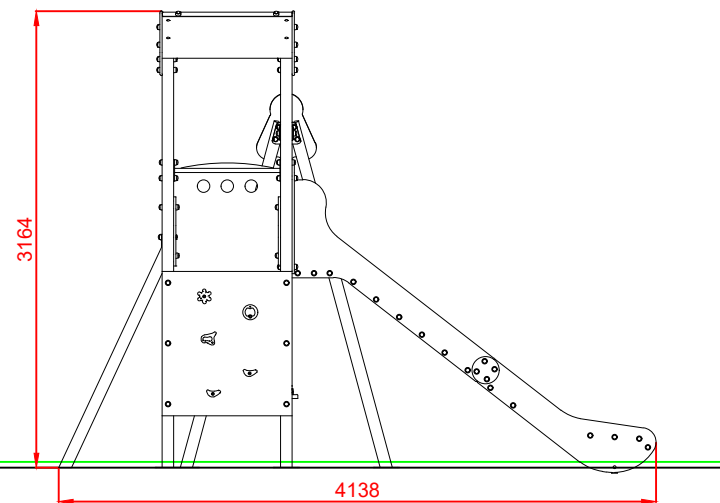
PERFIL IZQUIERDO
