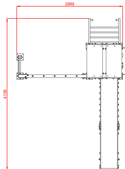
PLANTA
