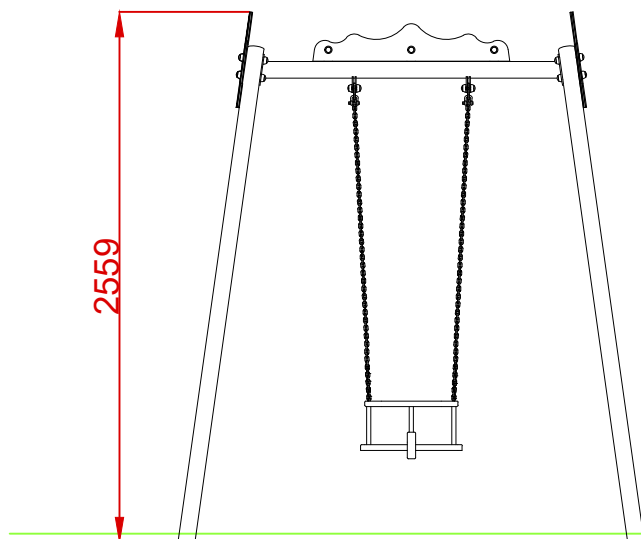
ALZADO
