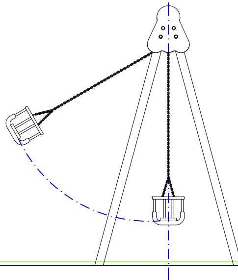
PERFIL
