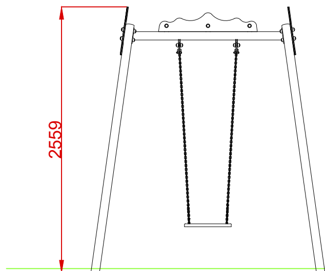
ALZADO
