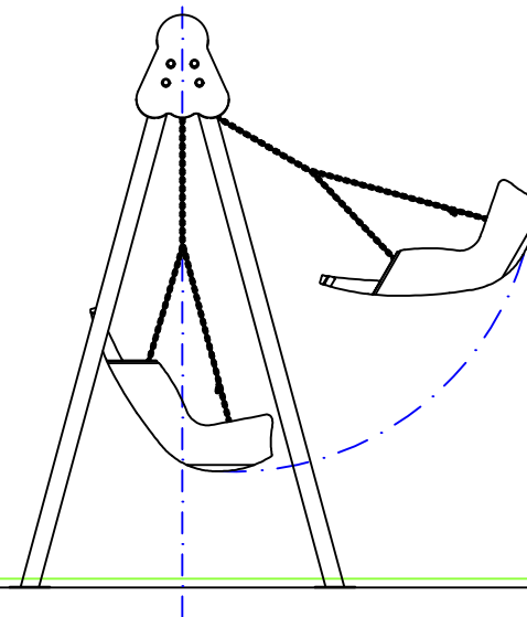
PERFIL
